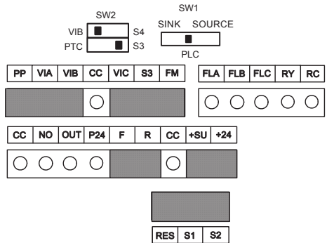
[Steuerklemmleiste]
