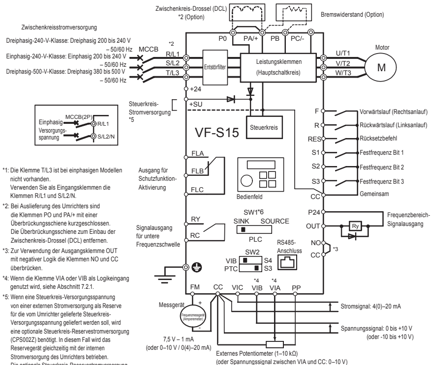
Anschlussdiagramm – negative Logik (SINK) (gemeinsam: CC)
